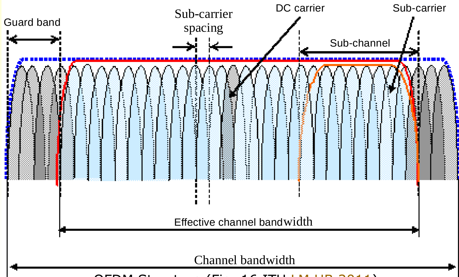
OFDM Structure (Fig. 16 ITU LM HB 2011 )
